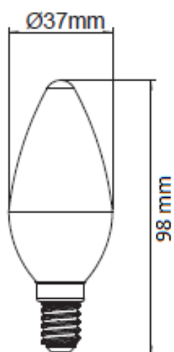
Rysunek techniczny:
